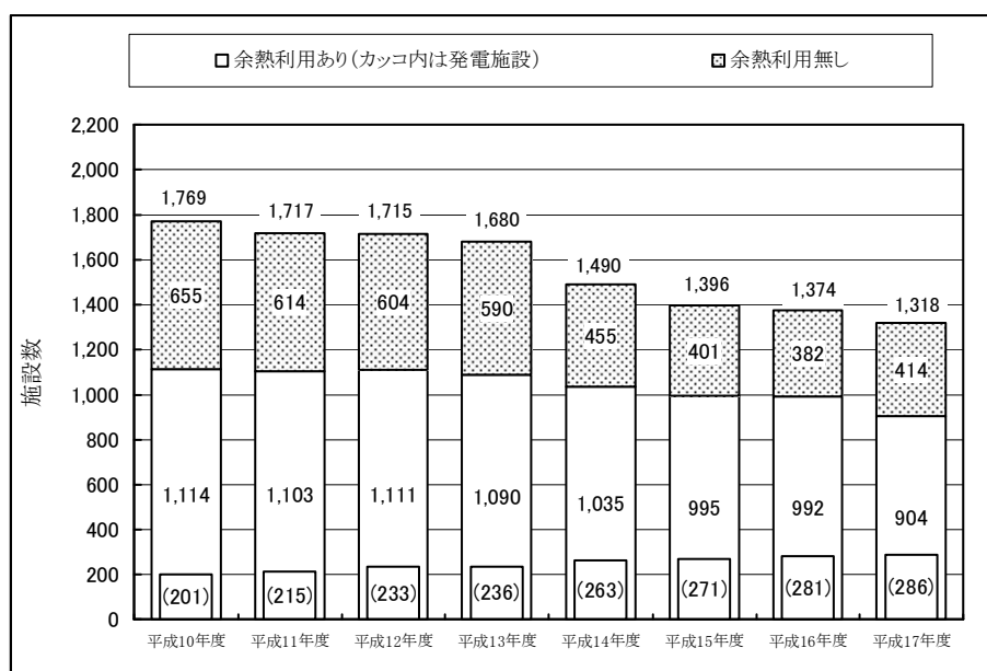
図－１３ ごみ焼却施設の余熱利用の推移
