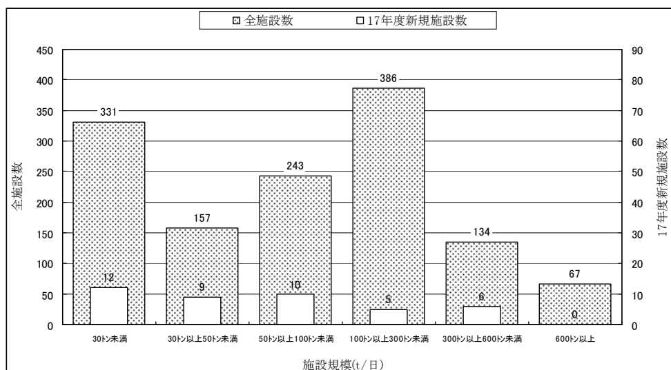
図－１２ ごみ焼却施設の規模別施設数
