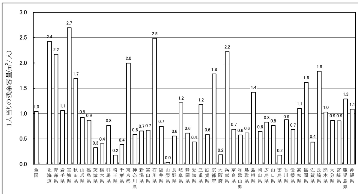
図－２１ 都道府県別の一人当たりの残余容量
