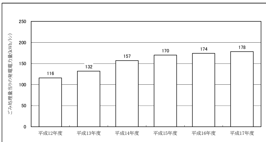
図－14 ごみ処理量当たりの発電電力量
