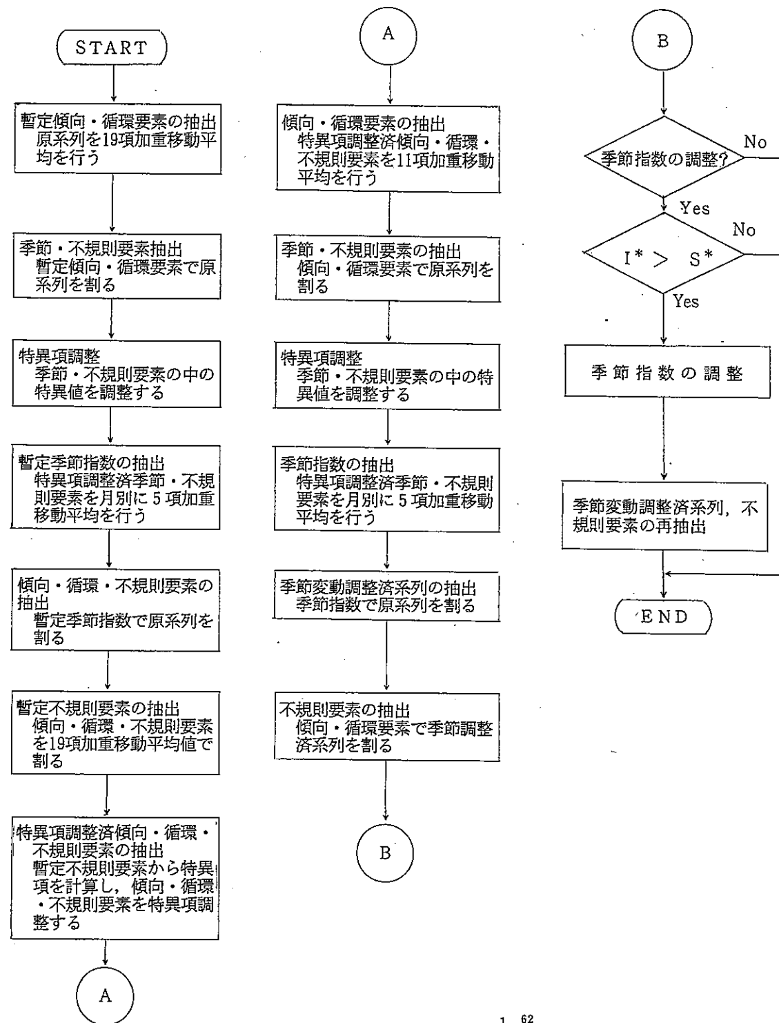
MITI法ⅢRのブロックチャート（分析計算の部分を除く）
