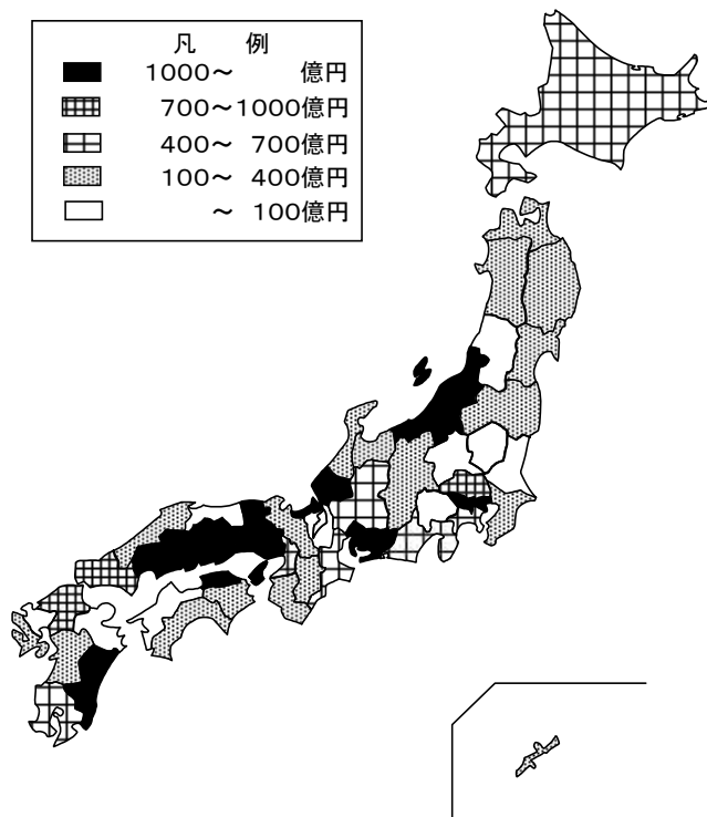
図一11 過去10年間都道府県別一般資産等被害累積額分布図（平成12年価格）
