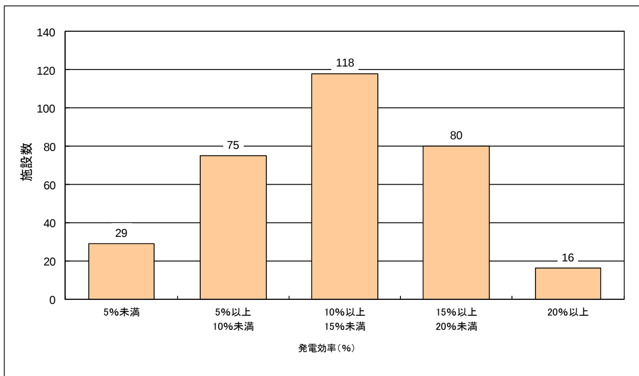
図－１４ ごみ焼却施設の発電効率別の施設数 注15)
