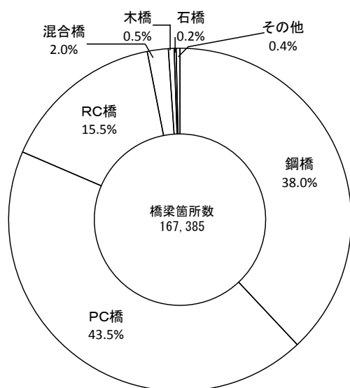
(イ) 橋種別橋梁箇所数比率
