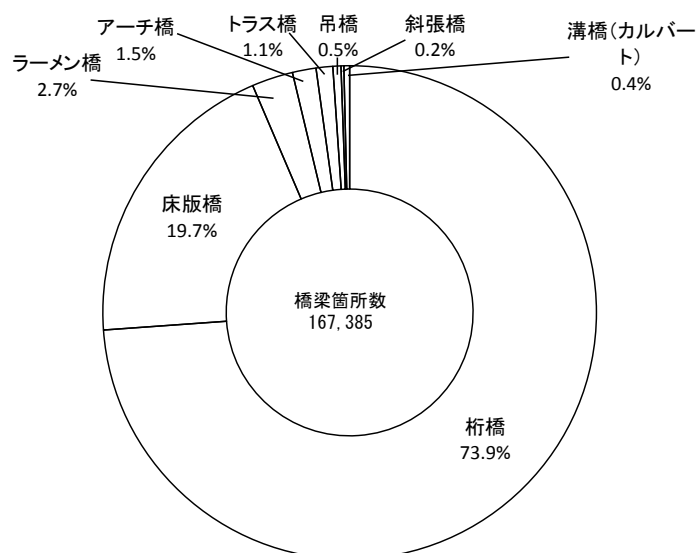
(ニ) 橋梁構造形式別橋梁箇所数比率
