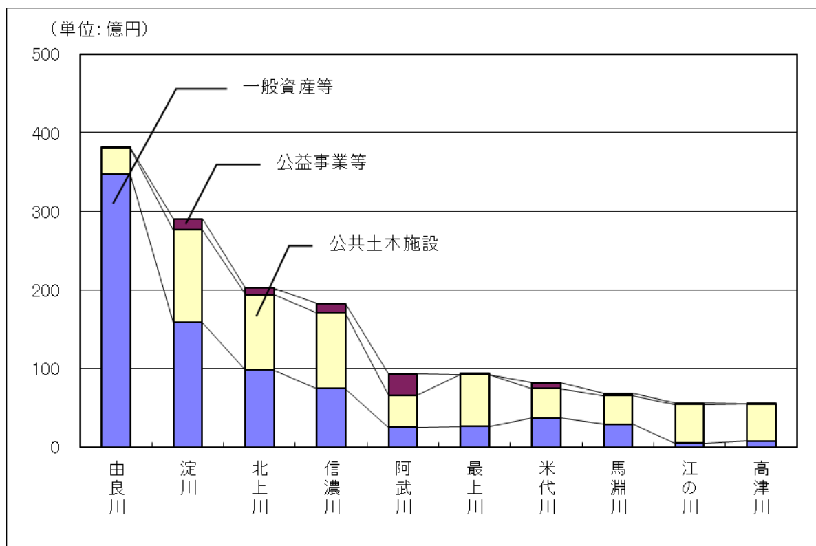
図－6 主要水系別水害被害額（被害額上位10水系）
