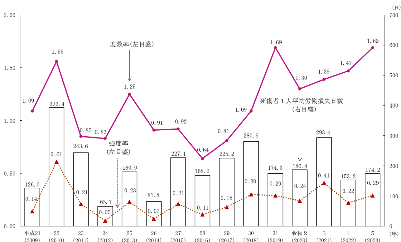
第3図 労働災害率及び死傷者1人平均労働損失日数の推移(総合工事業)
